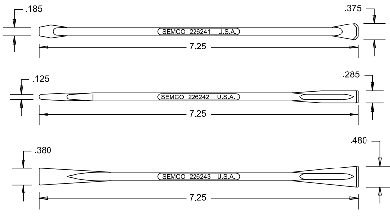
Spatula kit (all 3 spatulas) P/N 226244
