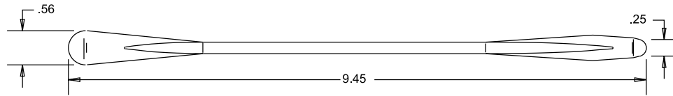
Spatula P/N 231349
